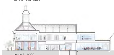
coupe A 1/200
